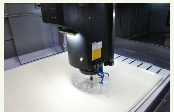
▷우성하이테크에 설치된 제조설비 ‘머시닝센터’
